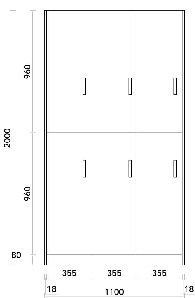
A柜立面图
