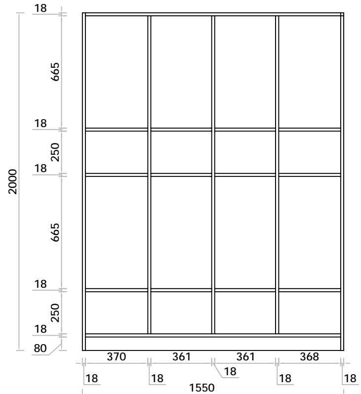
C柜结构图
