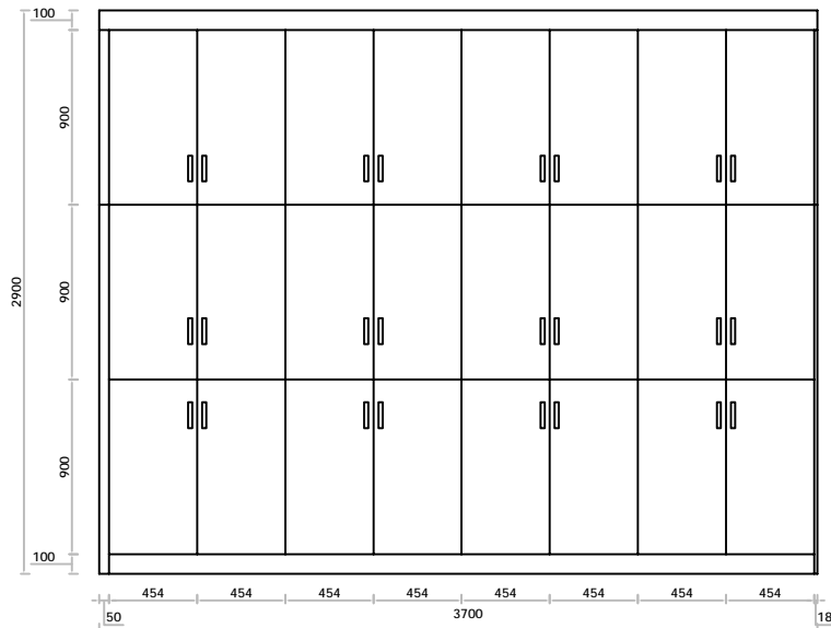
C柜立面图
