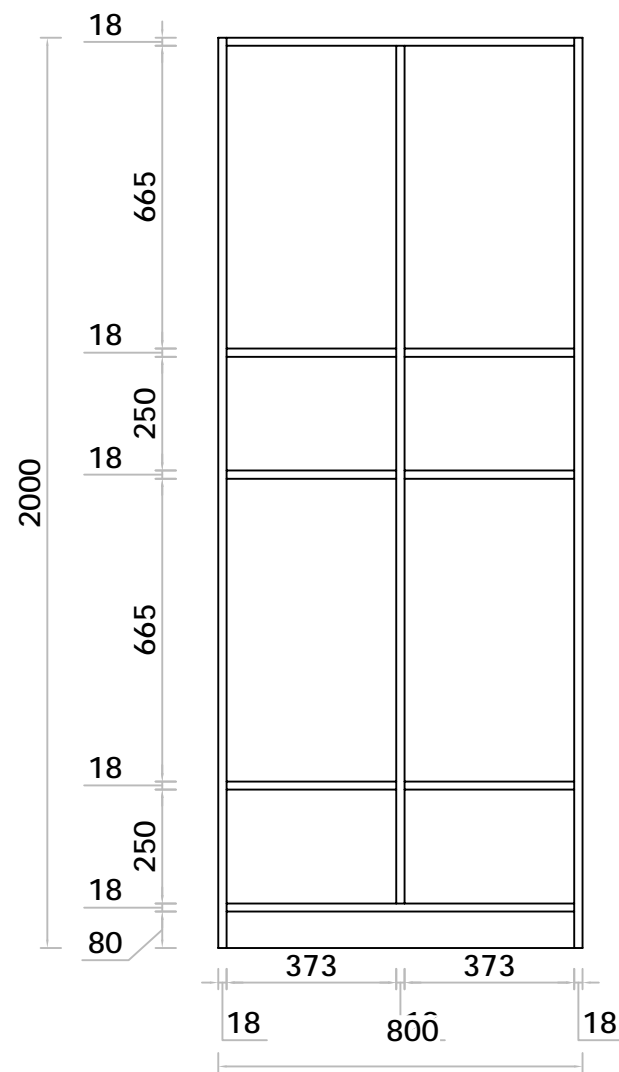
D柜结构图
