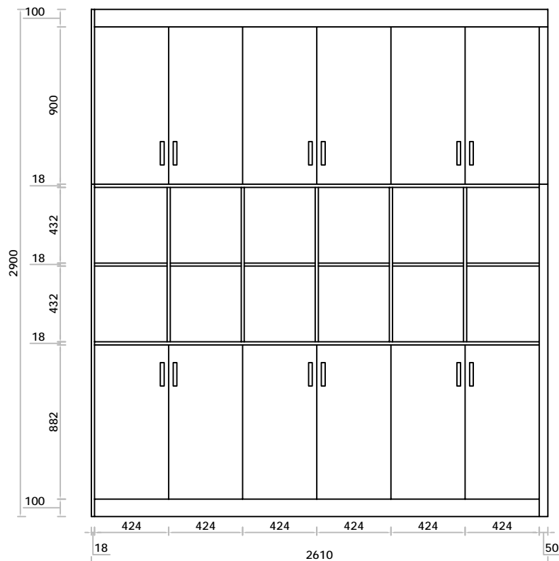
A柜立面图
