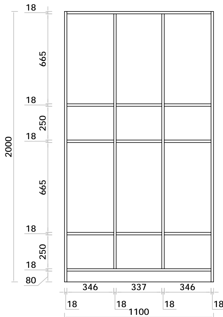
A柜结构图
