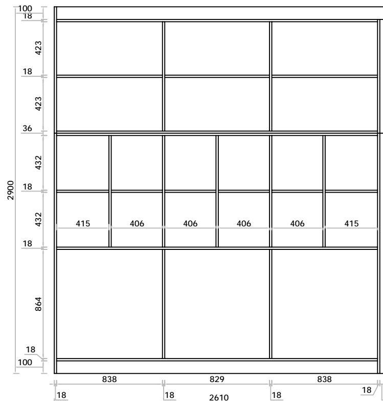
A柜结构图
