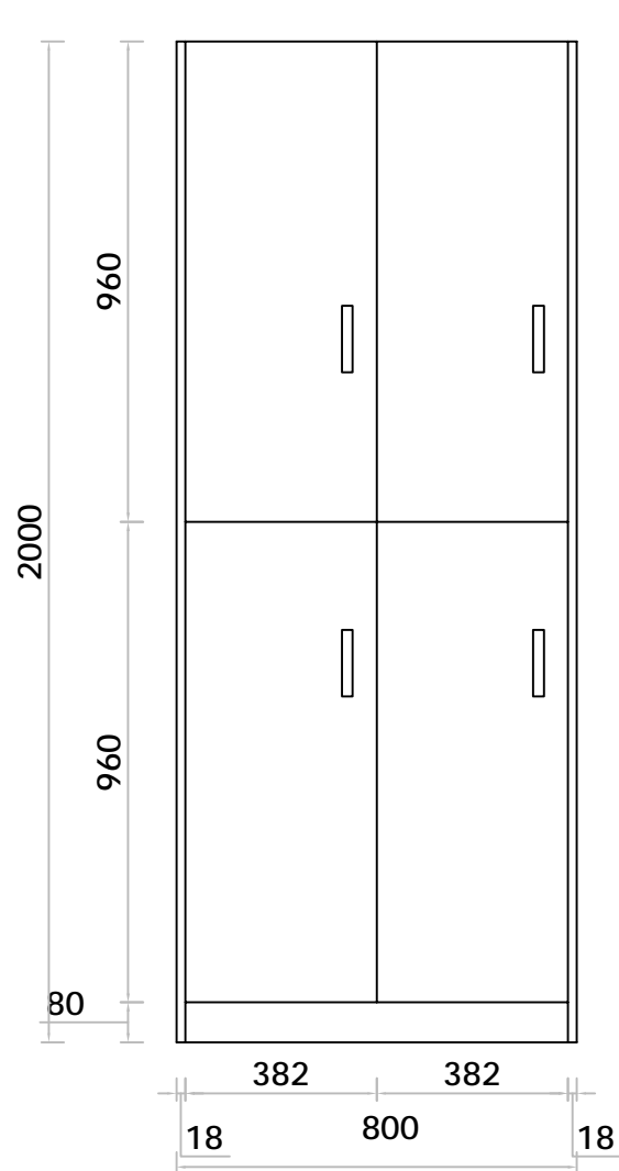
D柜立面图
