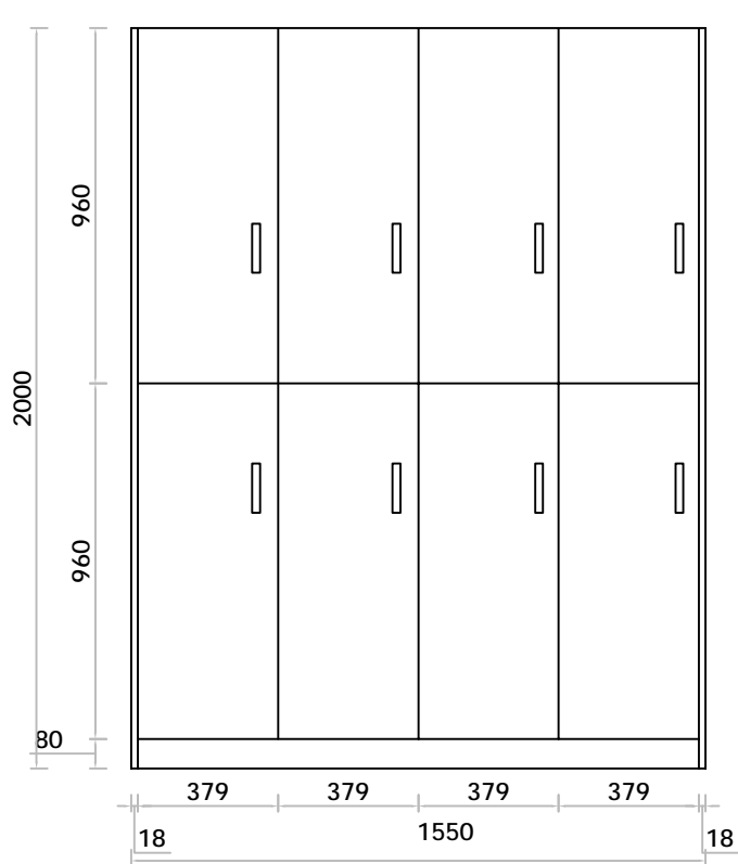
C柜立面图
